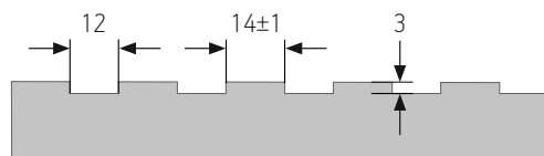
Сечение
